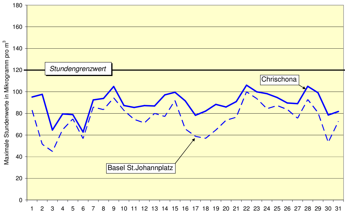
Ozon (O 3 ): Verlauf der täglichen maximalen Stundenwerte im März 2009
