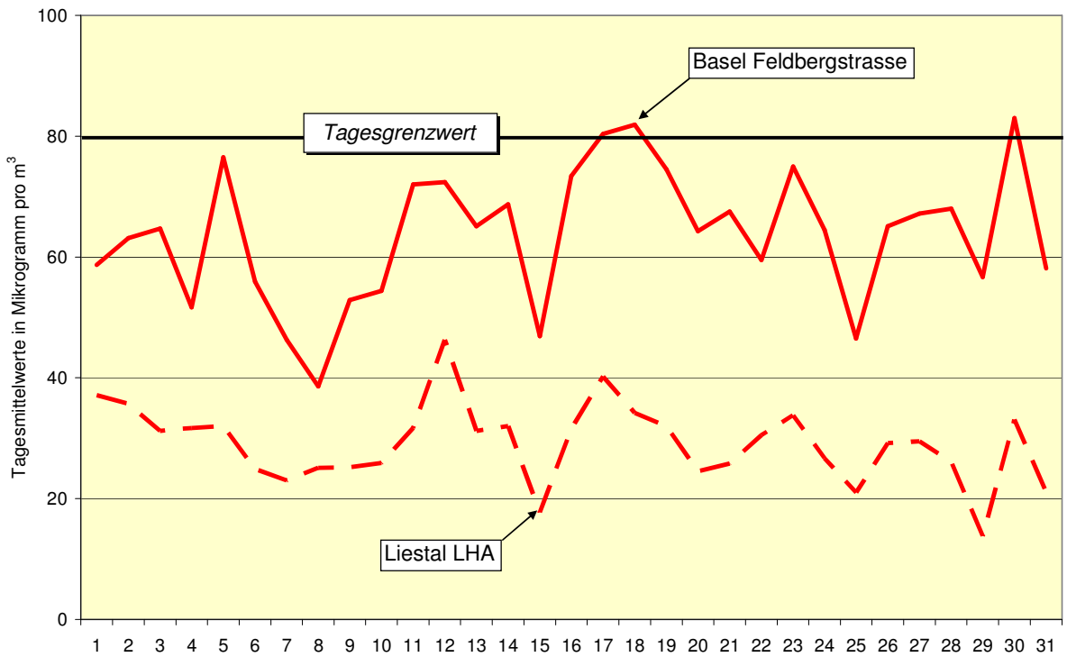
Stickstoffdioxid (NO 2 ): Verlauf der Tageswerte im März 2009
