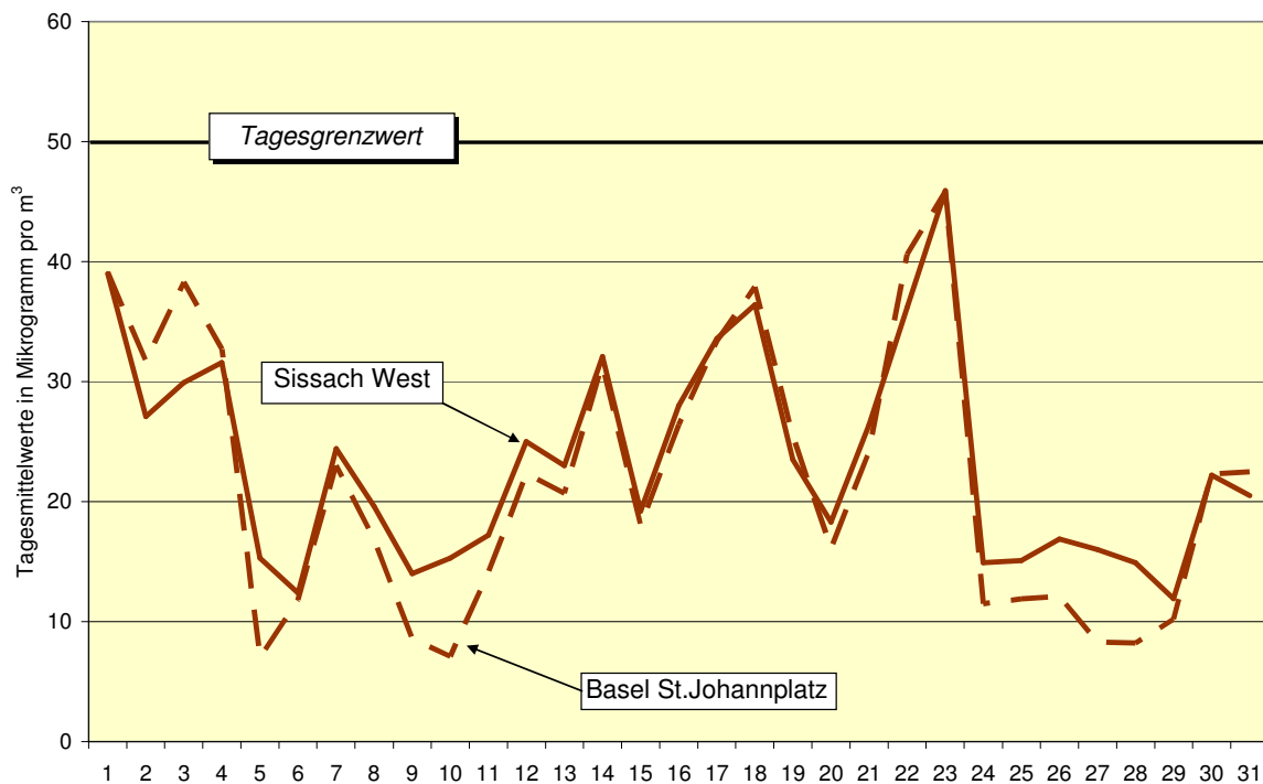
Feinstaub (PM10): Verlauf der Tageswerte im März 2009
